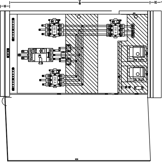
نمای جلو
